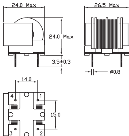
2 GROOVES BOBBIN:
