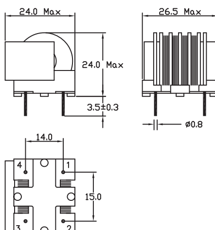
4 GROOVES BOBBIN:
