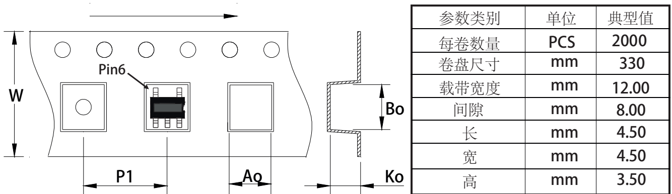
包装示意图
