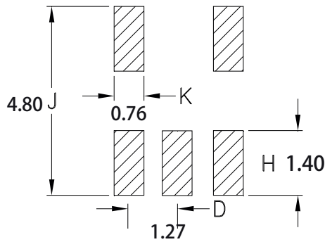
建议PCB布局图(mm)
